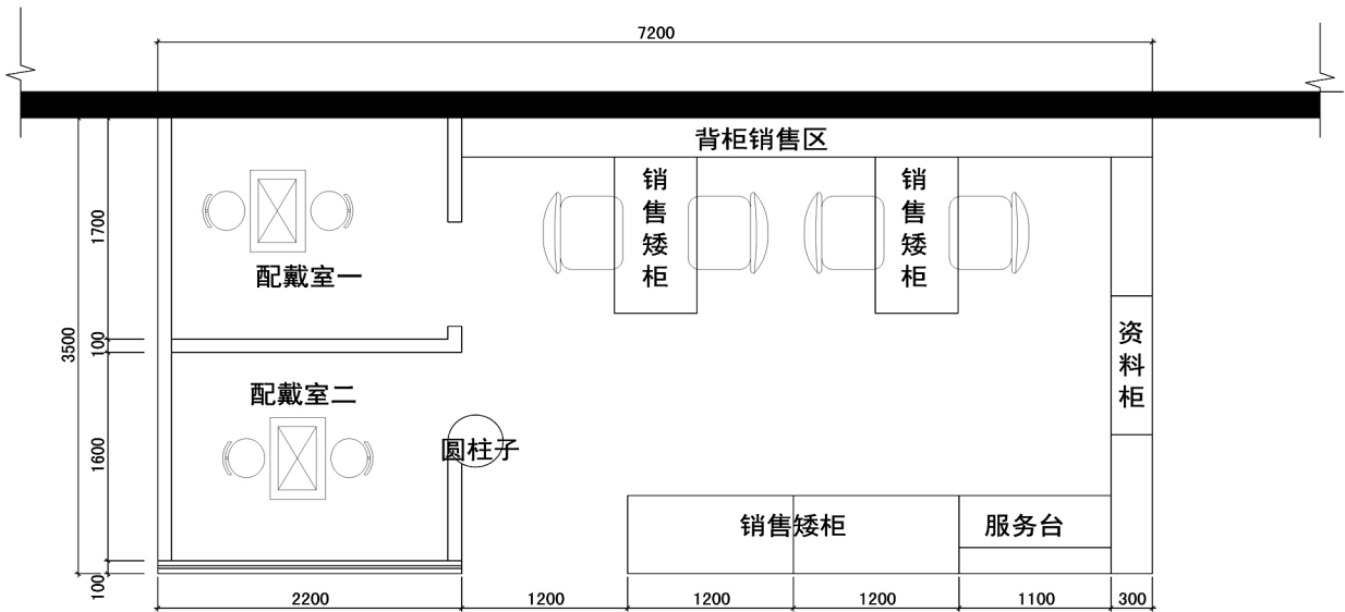
平面布置图
